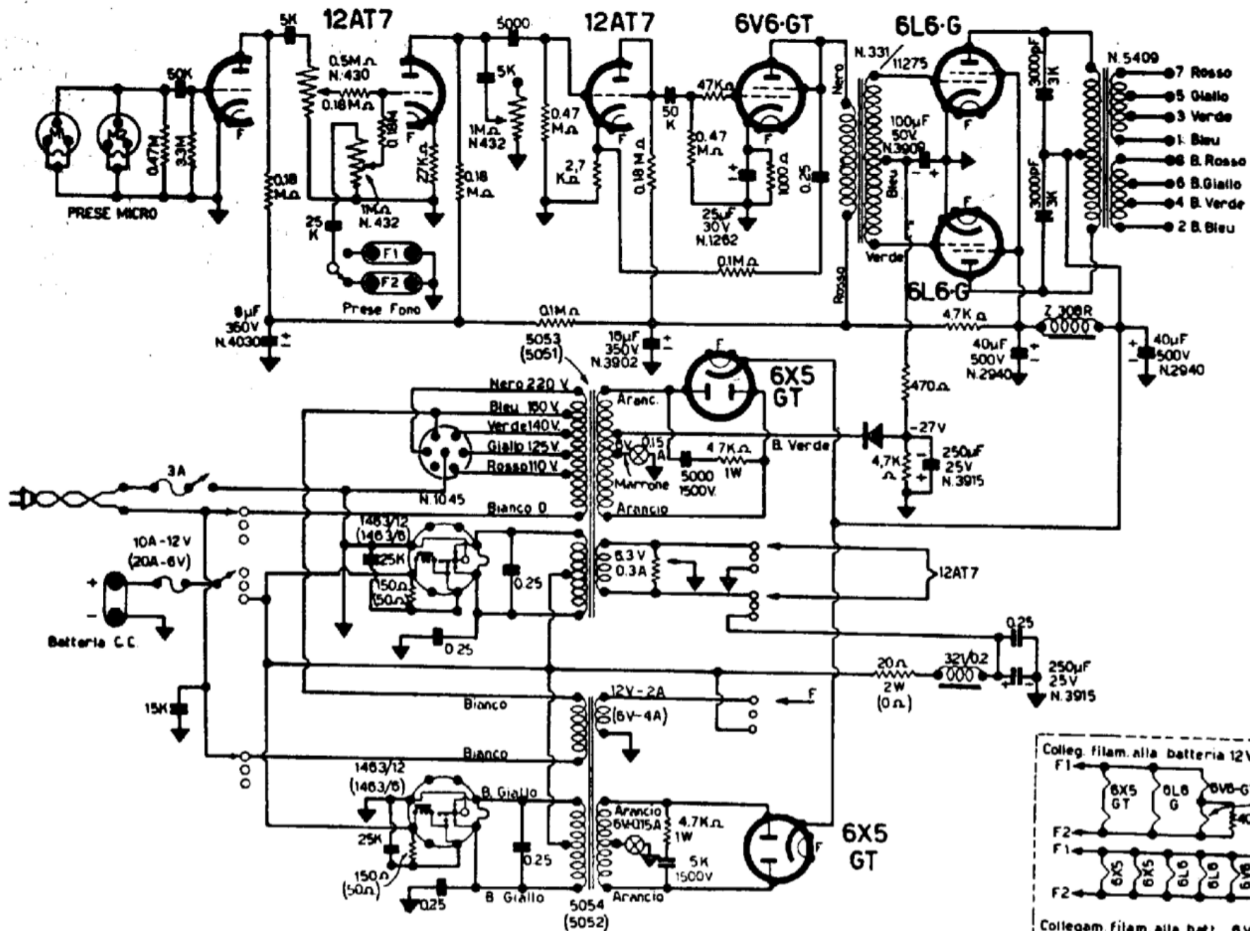
AMPLIFICATORE G. 229/12 (229/6)
